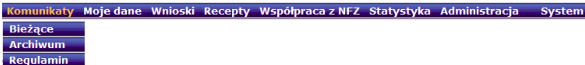
Rys. 4.1 Menu: Komunikaty
